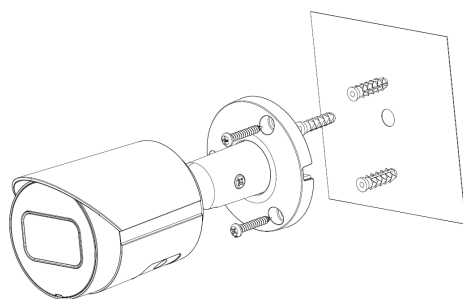
Vista detalhada VIP 3430 B G2
