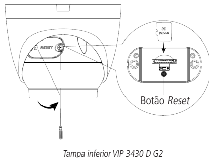
Tampa inferior VIP 3430 D G2
