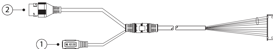
Cabo multifunções VIP 3430 B G2 e VIP 3430 D G2
