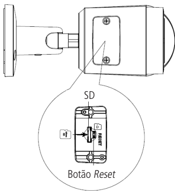
Tampa inferior VIP 3430 B G2
